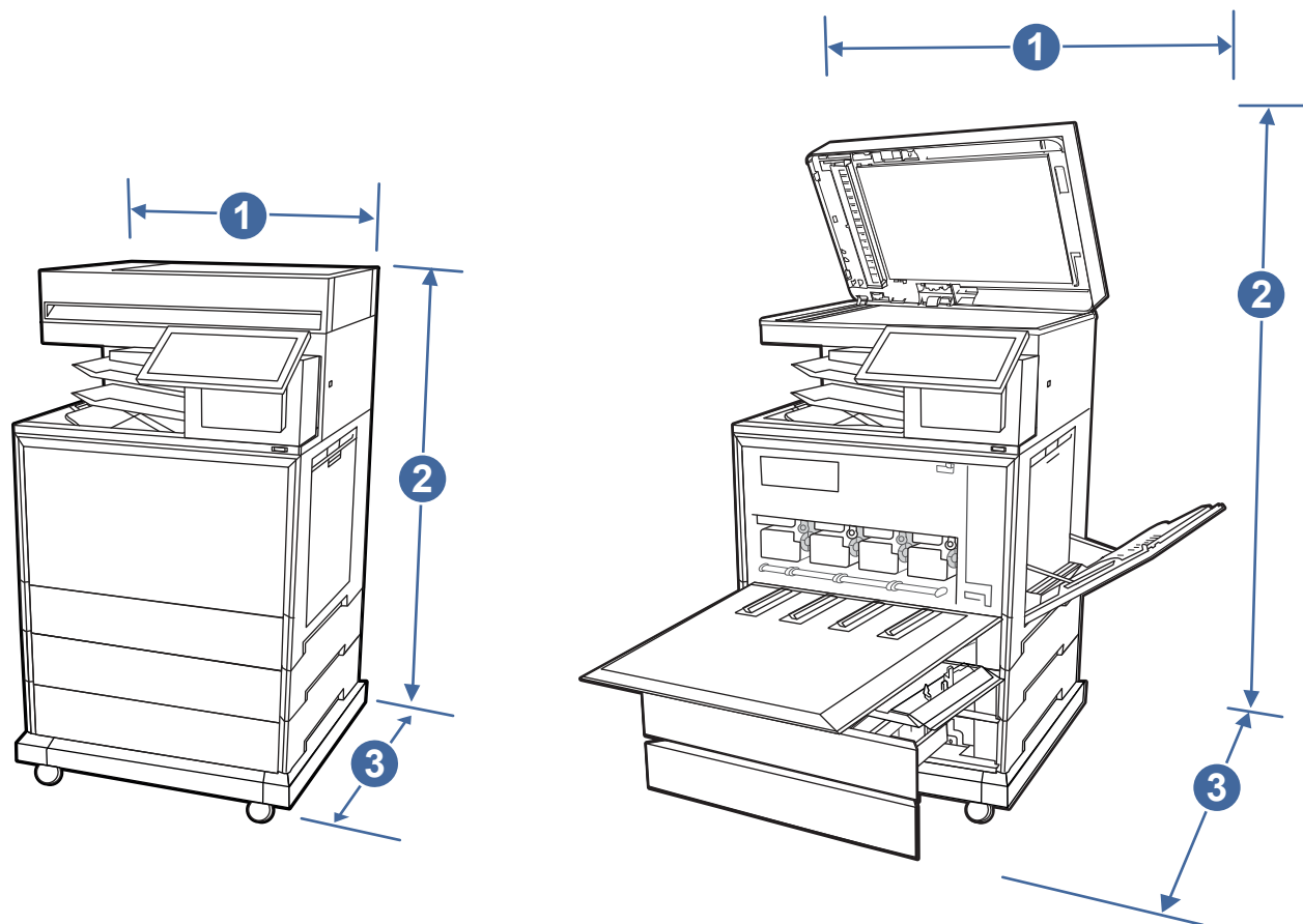
Rysunek 1-11 Wymiary drukarki (modele zfsw)
