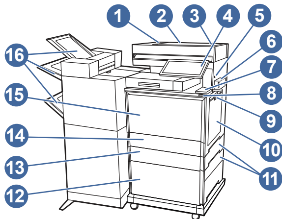
Rysunek 1-7 Widok drukarki z przodu - model zfw+
