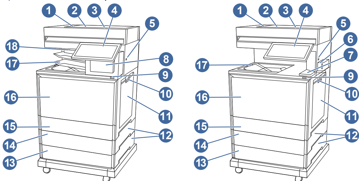
Rysunek 1-6 Widok drukarki z przodu - modele dn, zf i zfsw
