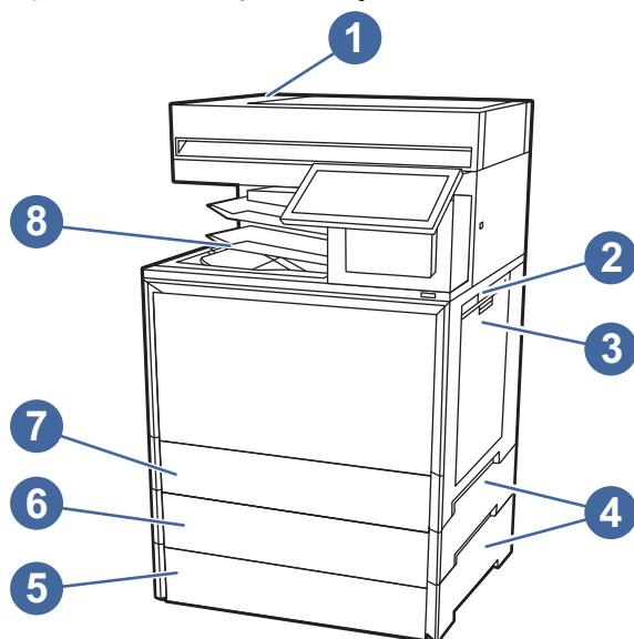
Rysunek 9-10 Miejsca zacięć - modele dn, zf i zfsw
