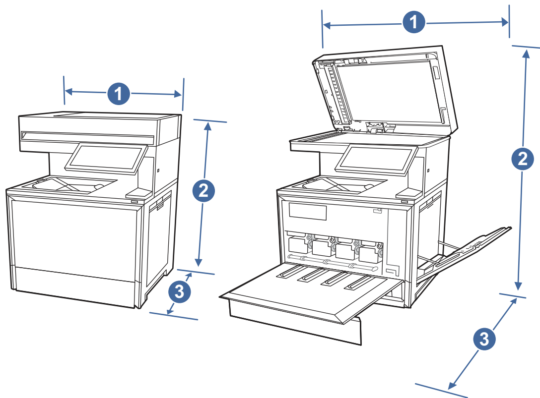
Rysunek 1-10 Wymiary drukarki (modele dn i zf)
