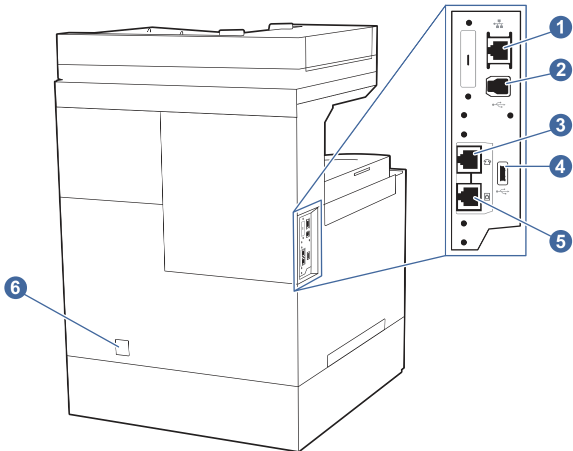
Rysunek 1-8 Widok drukarki z tyłu
