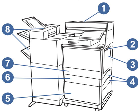
Rysunek 9-11 Miejsca zacięć - model zfw+
