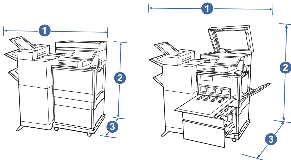
Rysunek 1-12 Wymiary drukarki (modele zfw+)
