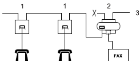
Rysunek 2: Zalecane połączenie gniazdek telefonów wewnętrznych
