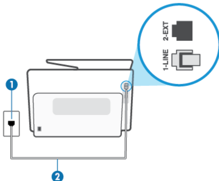
Rysunek 8-5 Widok drukarki z tyłu
