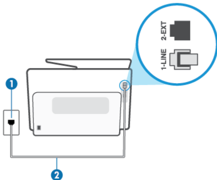
Rysunek 11-1 Widok drukarki z tyłu
