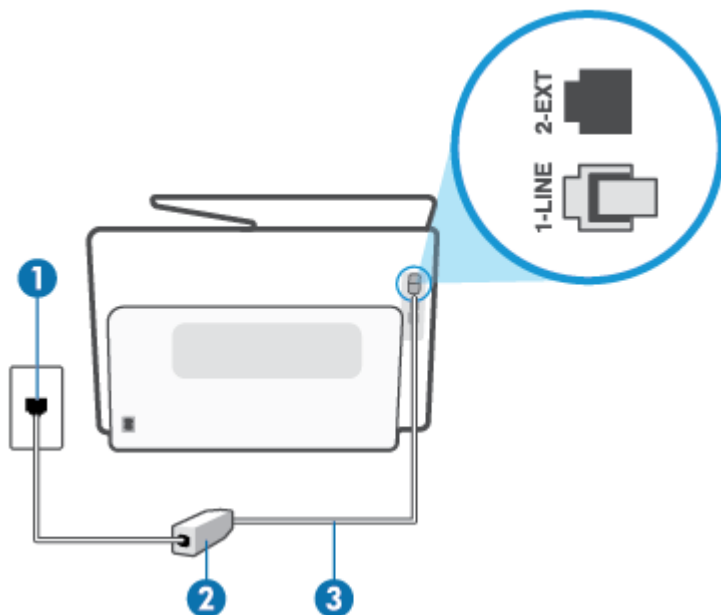
Rysunek 8-2 Widok drukarki z tyłu
