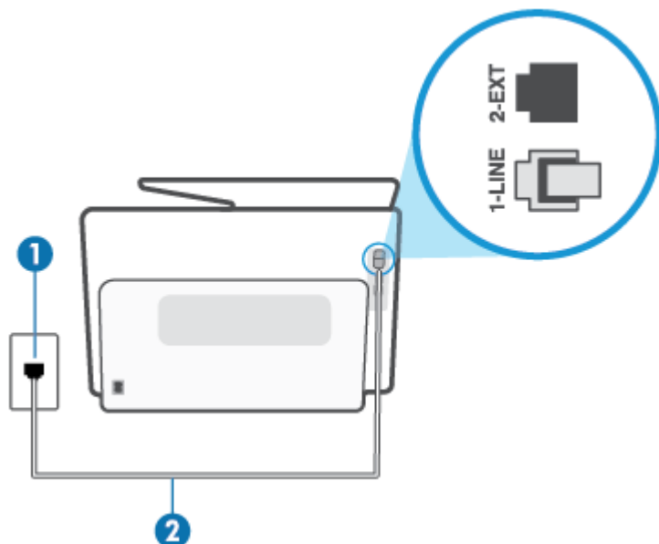
Rysunek 8-3 Widok drukarki z tyłu
