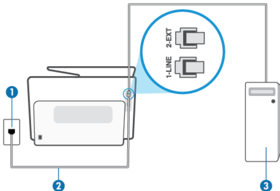
Rysunek 8-6 Widok drukarki z tyłu
